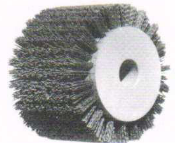
Schleifkornbürste Korn 60/80 Ø 150 Höhe 110 Bohrung 30 Ø 150 Höhe 120 Bohrung 30 Festo Ø 150 Höhe 90 Bohrung 30/16
